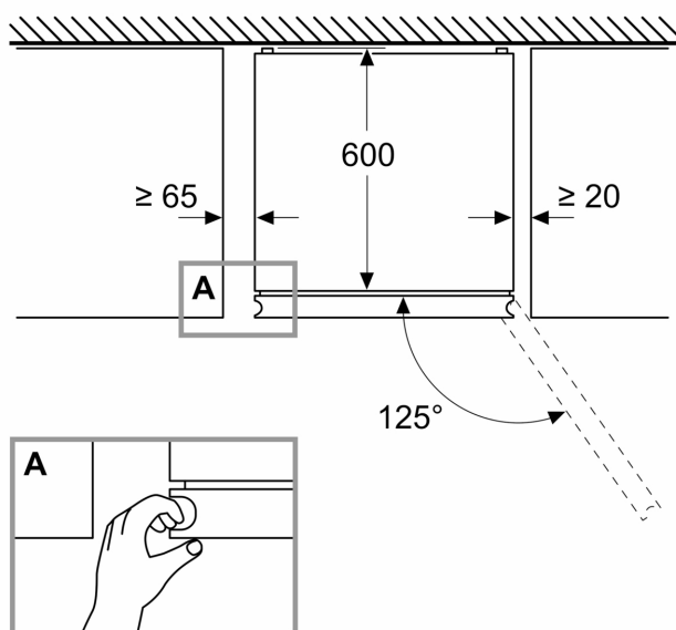
Mitat mm
