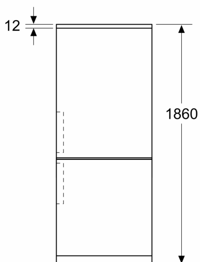
Mitat mm
